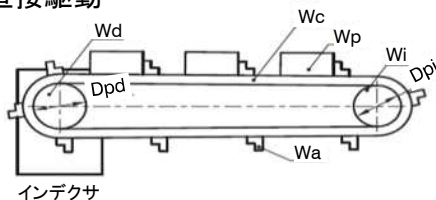
直接駆動
