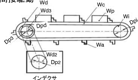
間接駆動
